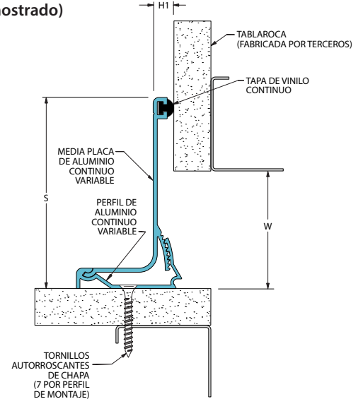
811-A09 Pared/Esquina Pared/Techo (2" (50mm) sistema mostrado)
