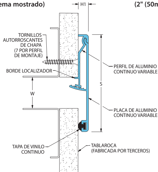
811-A07 Pared/Pared Techo/Techo (1" (25mm) sistema mostrado)
