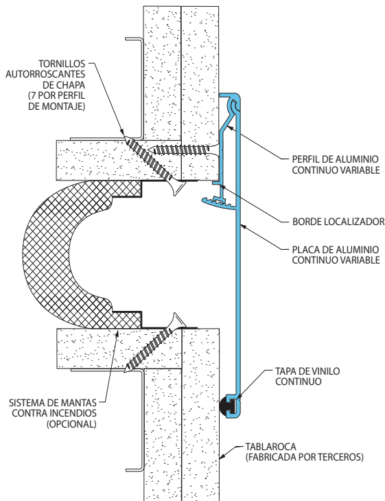
Sistema de Mantas Contra Incendios (811-A07-075 sistema mostrado)
