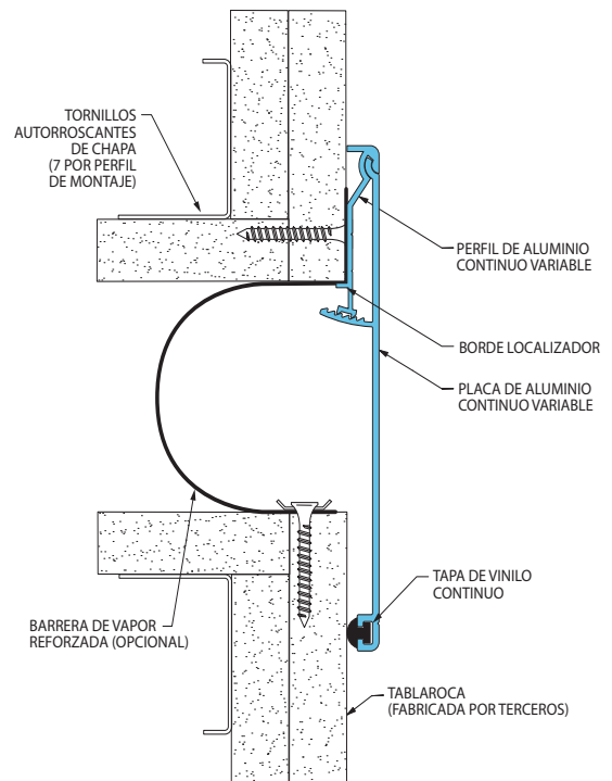
Sistema de Barreras de Vapor (811-A07-075 sistema mostrado)
